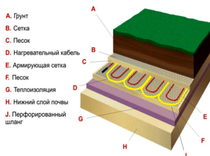
Рис. 2: Схема закладки системы подогрева и аэрации грунта
