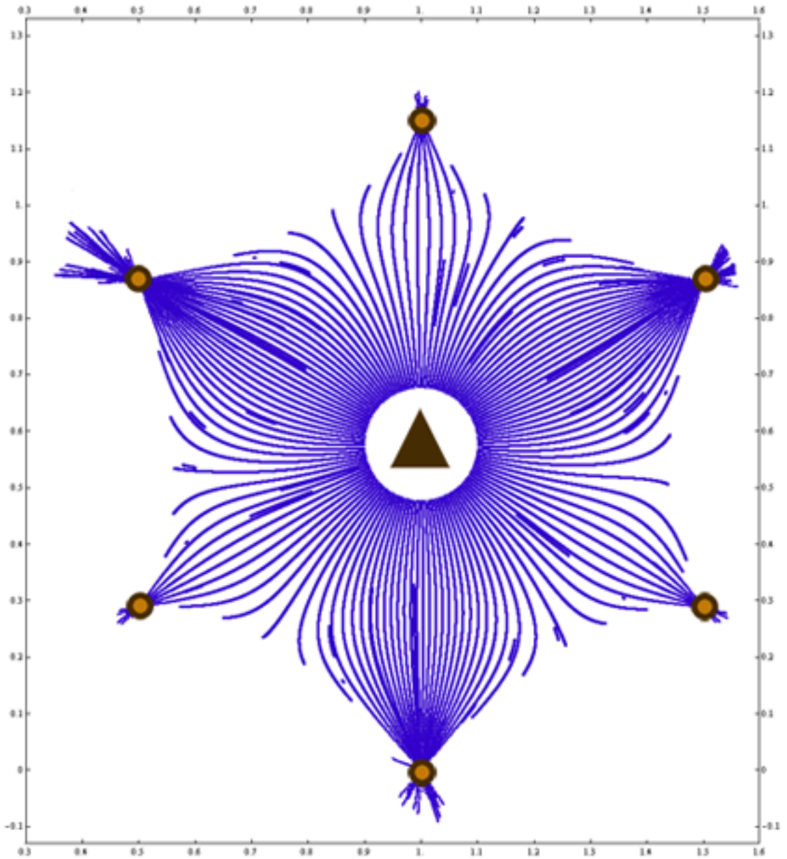
Рис. 2: Фронт заводнения для семиточечной схемы (момент прорыва). Время начала обводнения ( t ) - 750.
