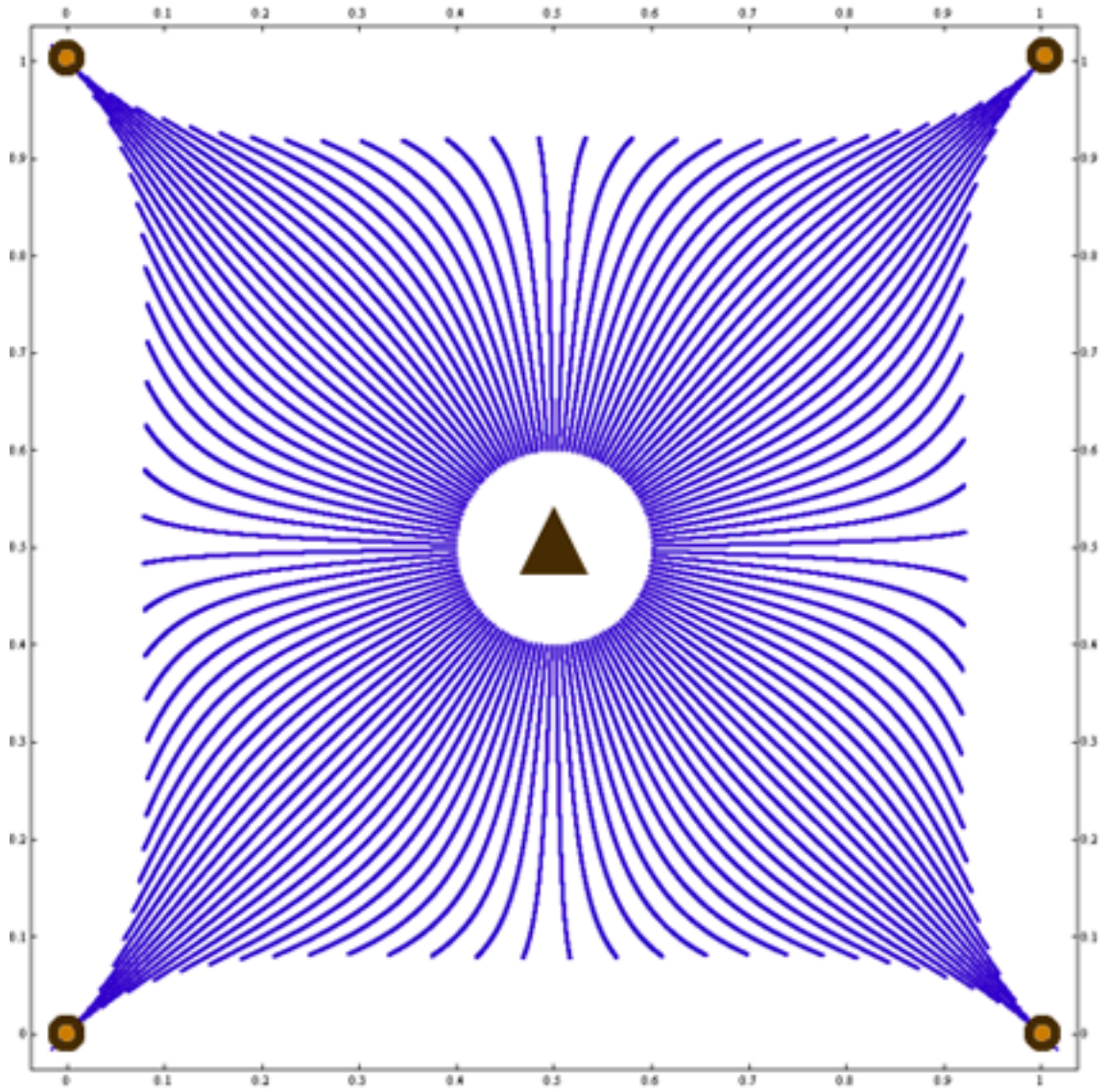
Рис. 1: Фронт заводнения для пятиточечной схемы (момент прорыва). Время начала обводнения (t) - 1100.
