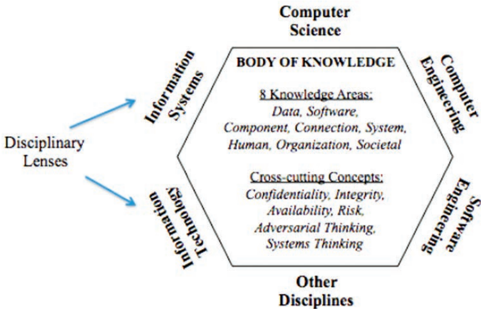
Рис. 9.2.2 CSEC-модель [73, С. 20].
