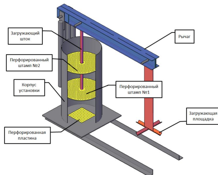
Рис. 1. Общий вид установки.
