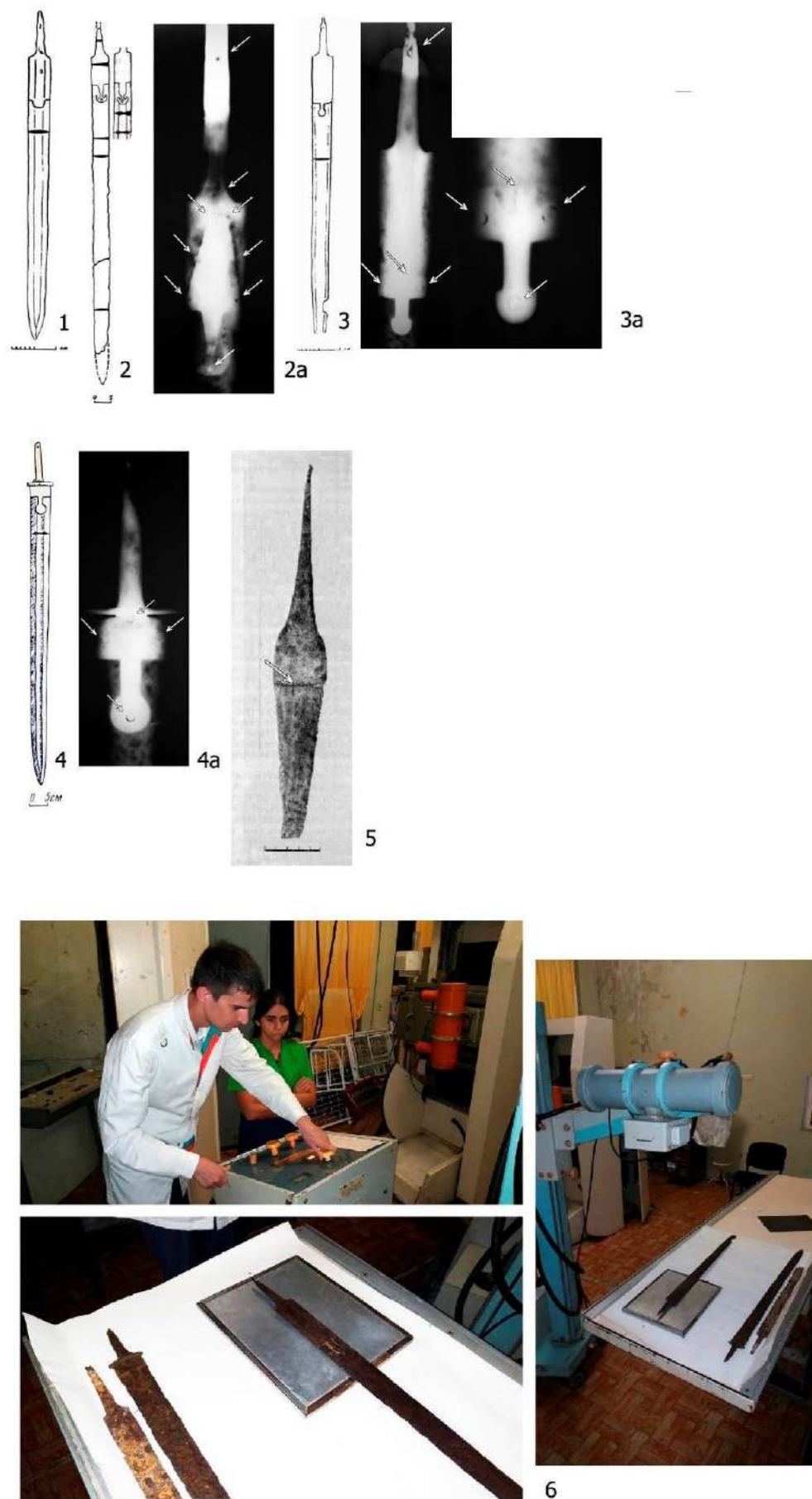
Рис. 1. Рентгенографическое исследование клинков
