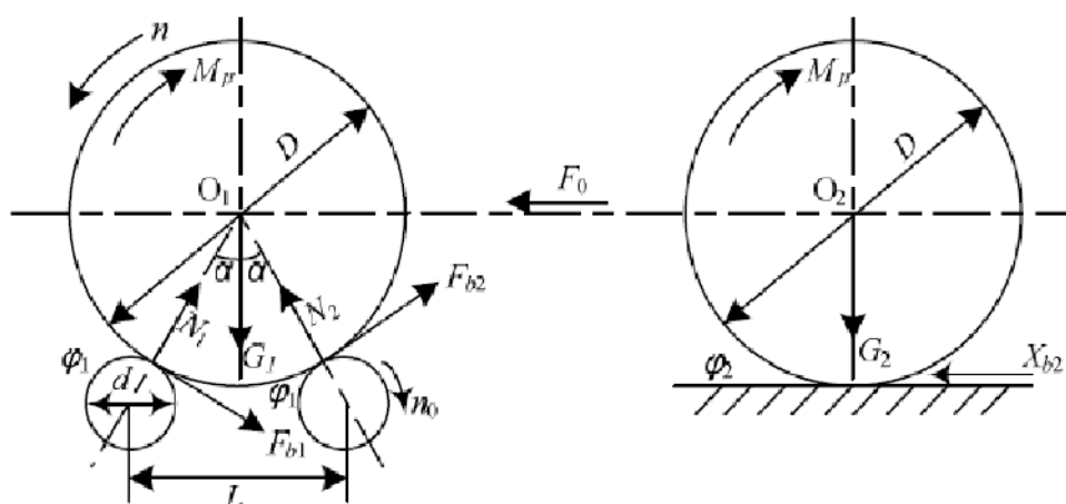
Рис. 2 Положение колеса на тормозном стенде.
