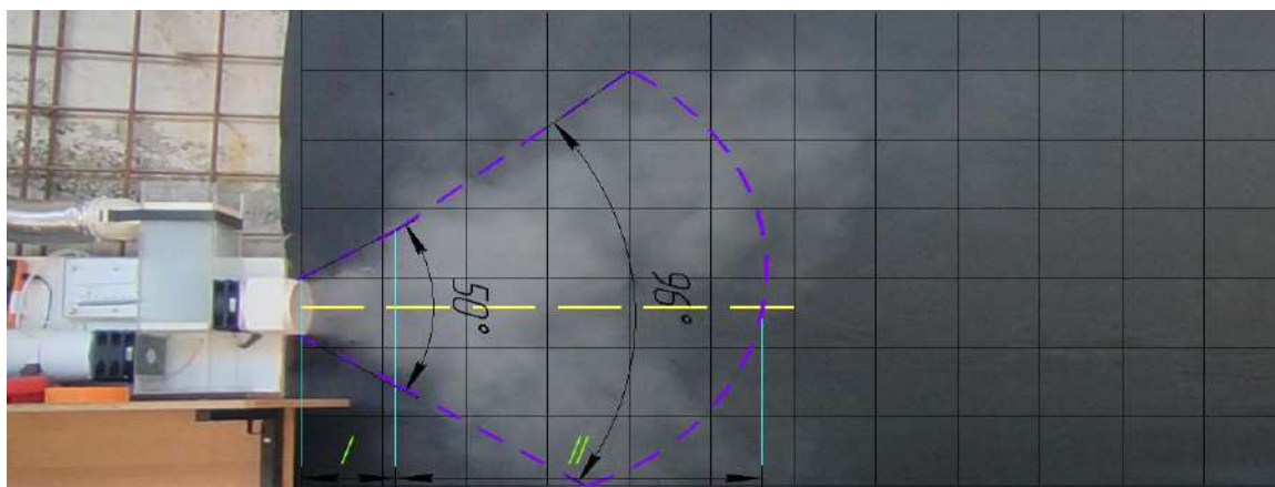
Рис. 3 Параметры распространения воздушного потока без спрямляющего аппарата: I – начальный участок; II – основной участок;
