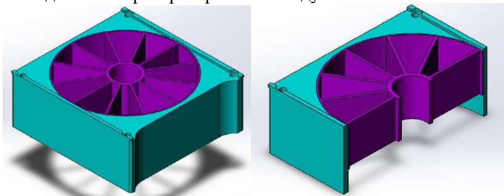
Рис. 2 Спрямляющий аппарат
