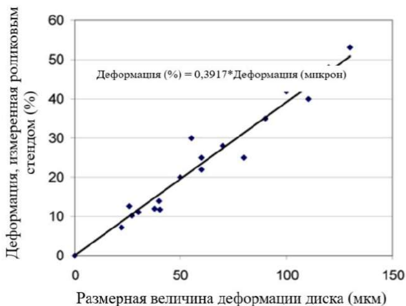
Рис. 1 Соотношение деформаций диска с параметрами, измеряемыми роликовым тормозным стендом.
