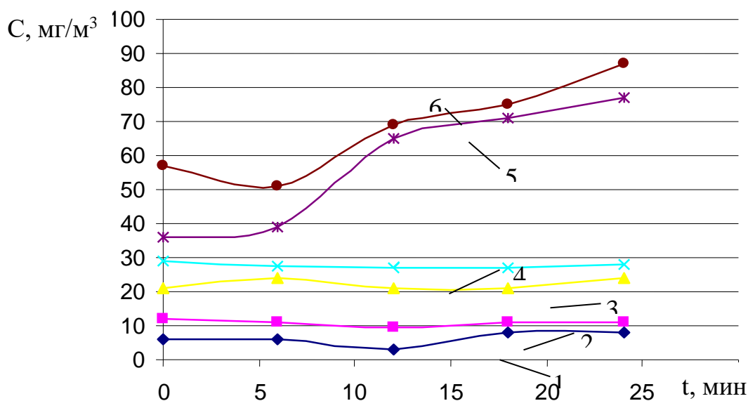
Рис.1 Изменение концентрации озона во времени при продувании через слой семян сахарной свеклы
