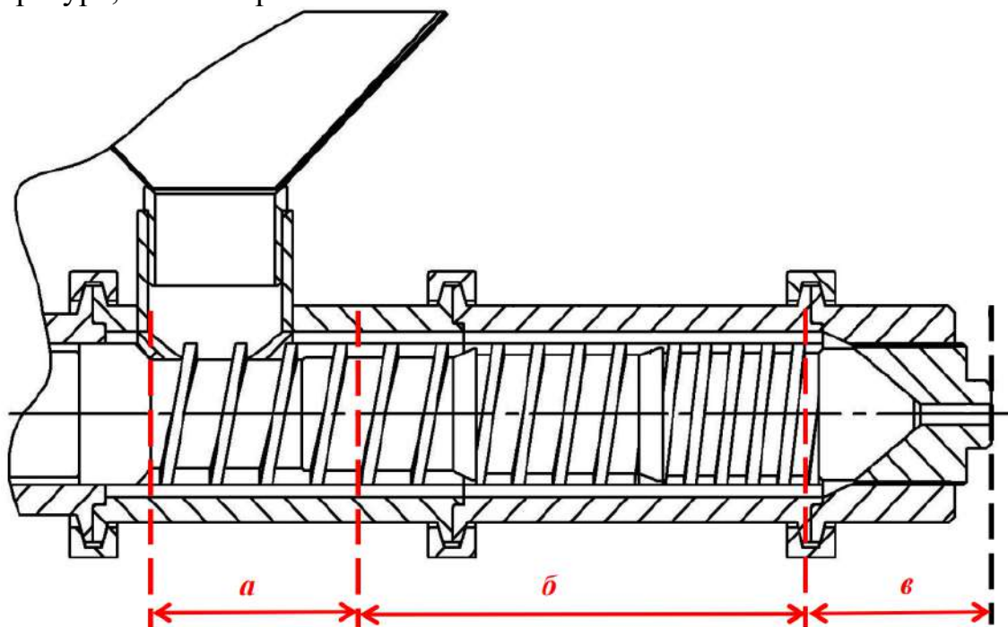
Рис. 3 Упрощенная схема шнекового экструдера
