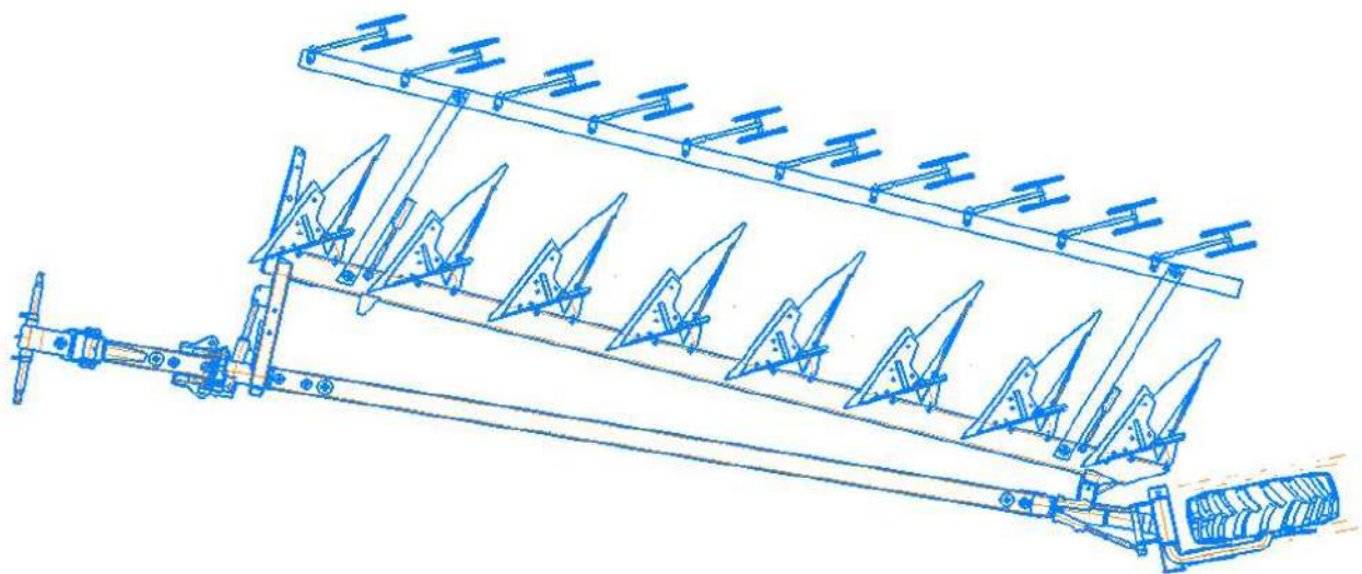
Рис. 1 Модернизированный оборотный плуг Gregoire Besson SP8
