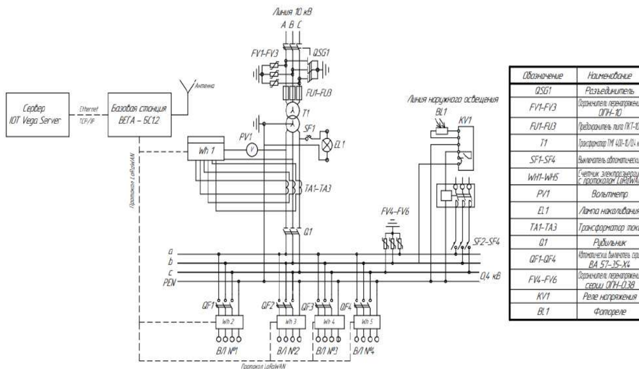
Рис.1 Структурная схема учета электроэнергии
