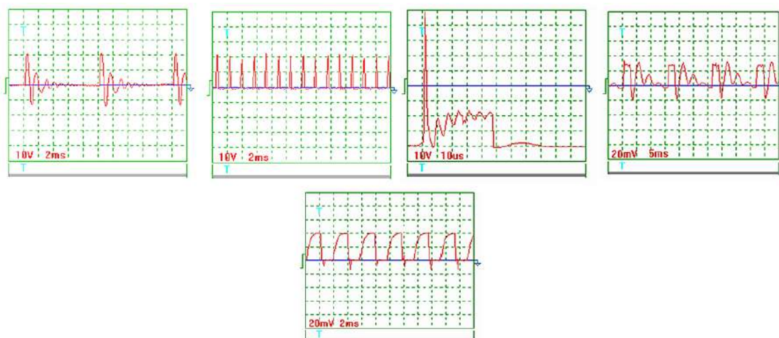
Рис. 4 Слева направо: Осциллограмма на аноде VS1, f=100 Гц (делитель осциллографа кратен 1 \times 10 ), Осциллограмма на коллекторе транзистора, f=600 Гц (делитель осциллографа кратен 1 \times 10 ), Осциллограмма на коллекторе транзистора VT1, f=600 Гц (делитель осциллографа кратен 1 \times 10 ) Осциллограмма формы тока, f=60 Гц (делитель осциллографа кратен 1 \times 10 ), Осциллограмма формы тока, f=318 Гц (делитель осциллографа кратен 1 \times 10 ).
