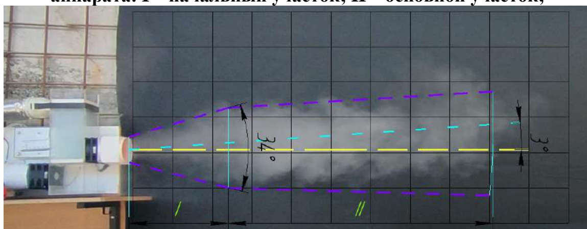
Рис. 4 Параметры распространения воздушного потока со спрямляющим аппаратом: I – начальный участок, II – основной участок
