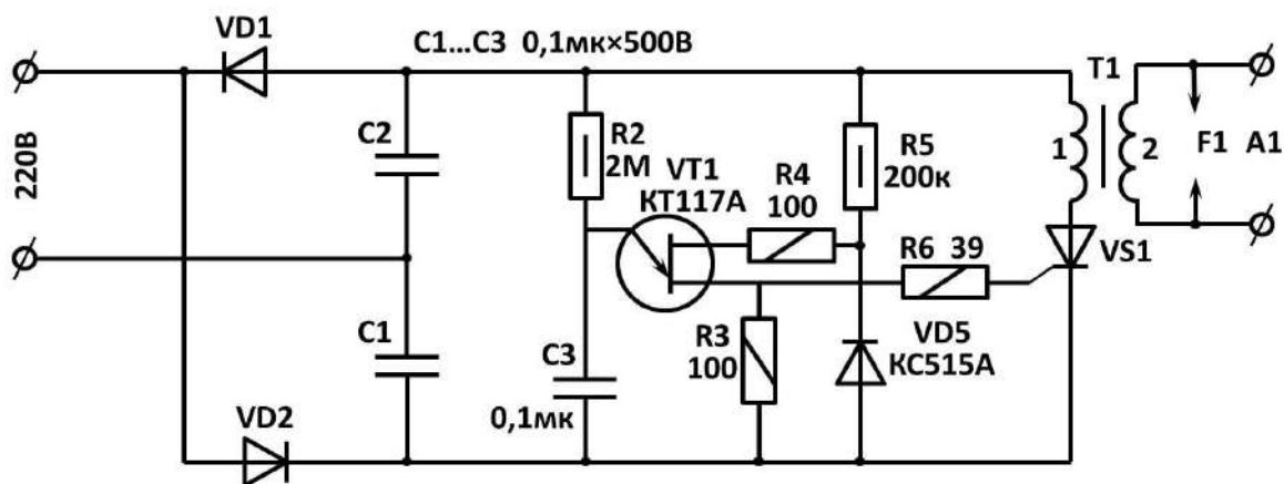
Рис. 1 Существующая принципиальная электрическая схема электроозонатора
