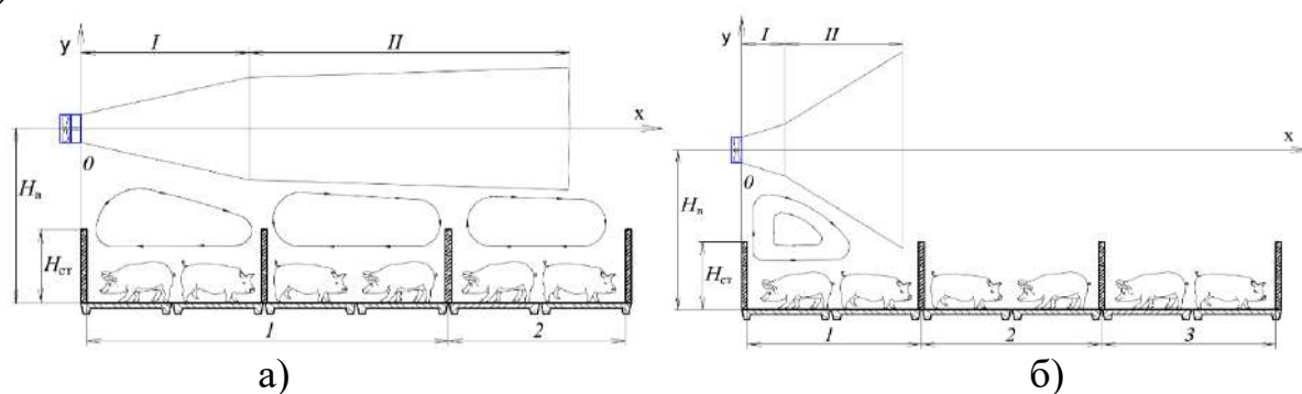
Рис.1 Типы струй: а – выровненная; б – закрученная;
