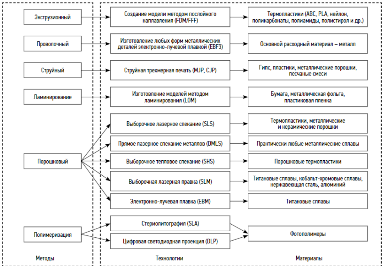
Рис. 1 Основные методы, технологии и материалы, применяемые в 3D-печати
