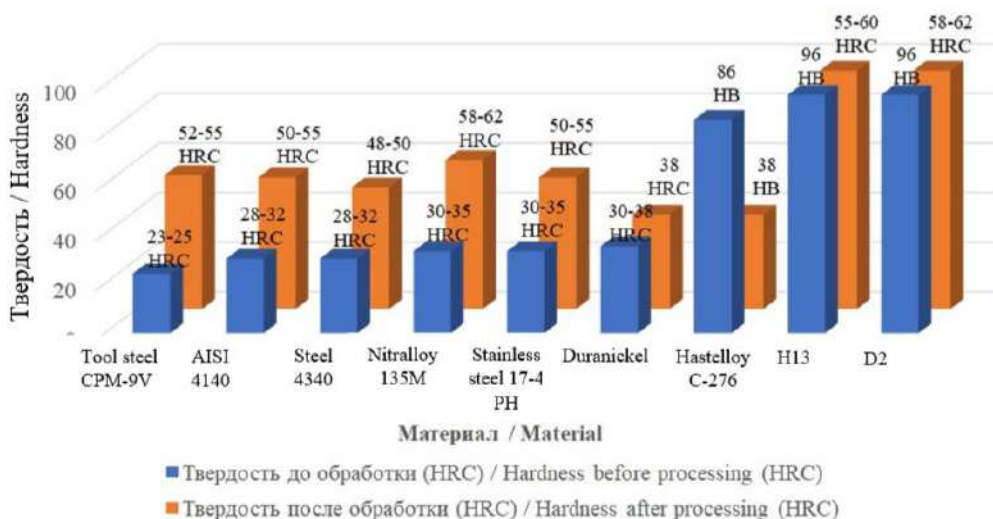
Рис.1 Материалы и их твердость, применяемые для изготовления шнековых рабочих органов
