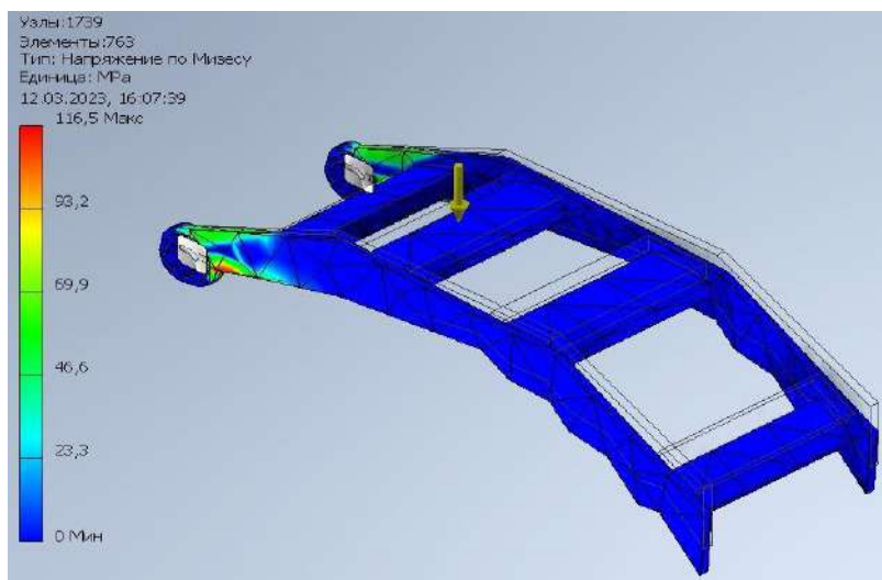
Рис.2 Прочностной расчет конструкции дополнительного захвата
