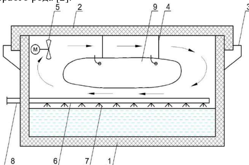
Рис. 1 Аппарат для охлаждения пищевых продуктов в газо-воздушной среде сублимирующего диоксида углерода
