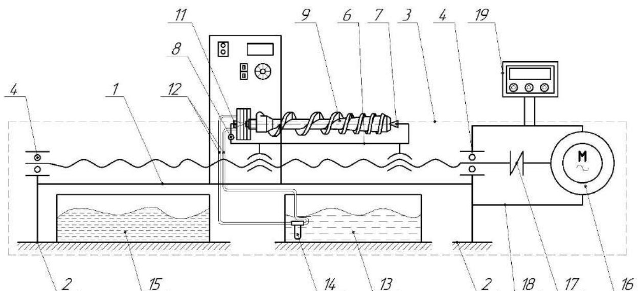
Рис. 1 Схема устройства для восстановления и упрочнения шнеков экструдеров диффузионным борированием в обмазках сверхвысокочастотным нагревом (заявка патента на изобретение № 2024108437): 1 – станина установки; 2 – опоры; 3 – перемещающее устройство; 4 – подшипниковый узел; 5 – главный винт; 6 – стол; 7 – БРС; 8 – БРС с подключенным откидывающим устройством; 9 – шнек; 10 – преобразователь частоты; 11 – индукционный нагреватель; 12 – трубопроводы; 13 – резервуар с охлаждающей жидкостью; 14 – погружной насос; 15 – резервуар с маслом; 16 – шаговый электродвигатель; 17 – соединительная муфта; 18 – подрамник; 19 – панель управления
