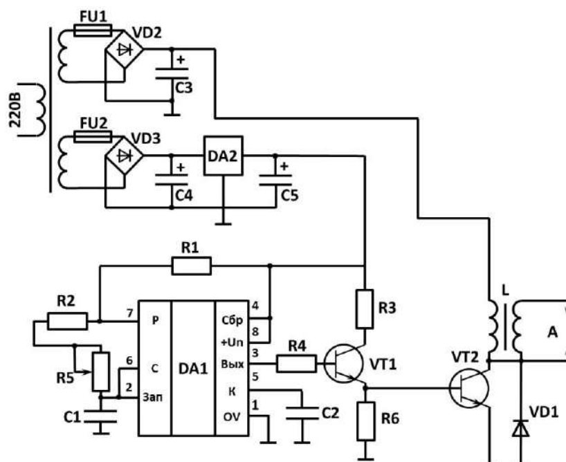
Рис.2 Разработанная принципиальная электрическая схема электроозонатора
