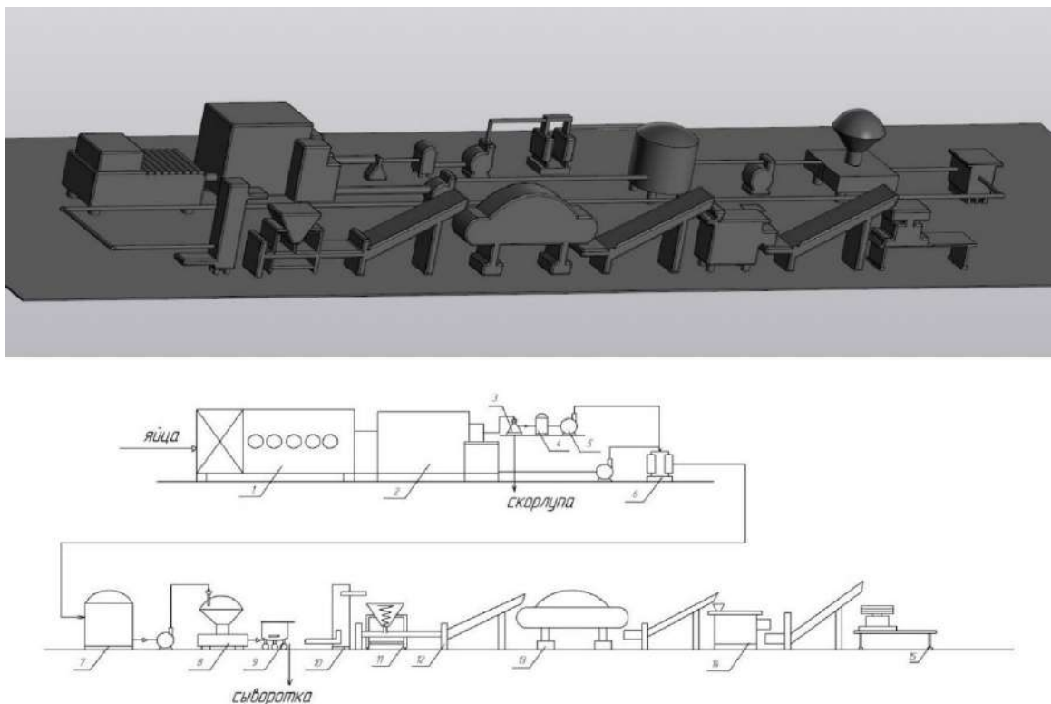
Рис. 1 Линия производства коагулированного яичного меланжа
