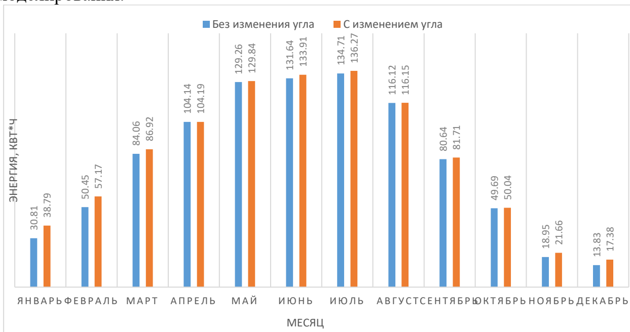
Рис.2 График генерации СФУ в течении года
