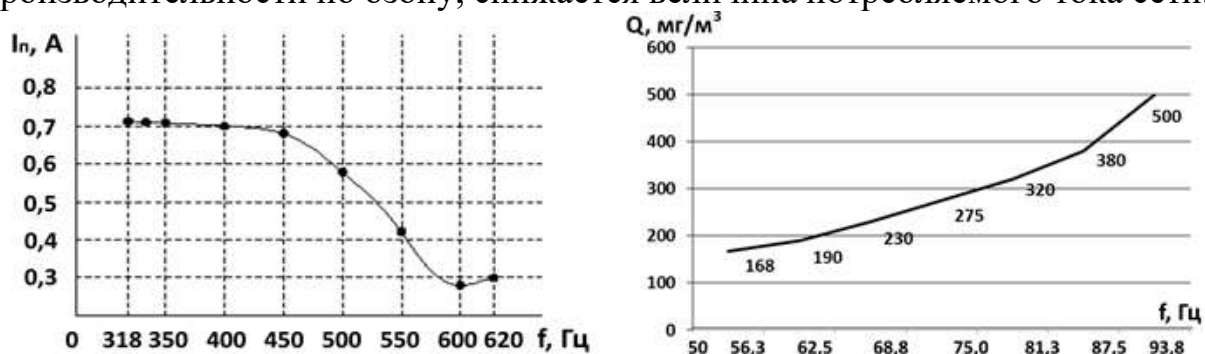
Рис. 3 Зависимость потребляемого тока от частоты, Зависимость концентрации озона от частоты
