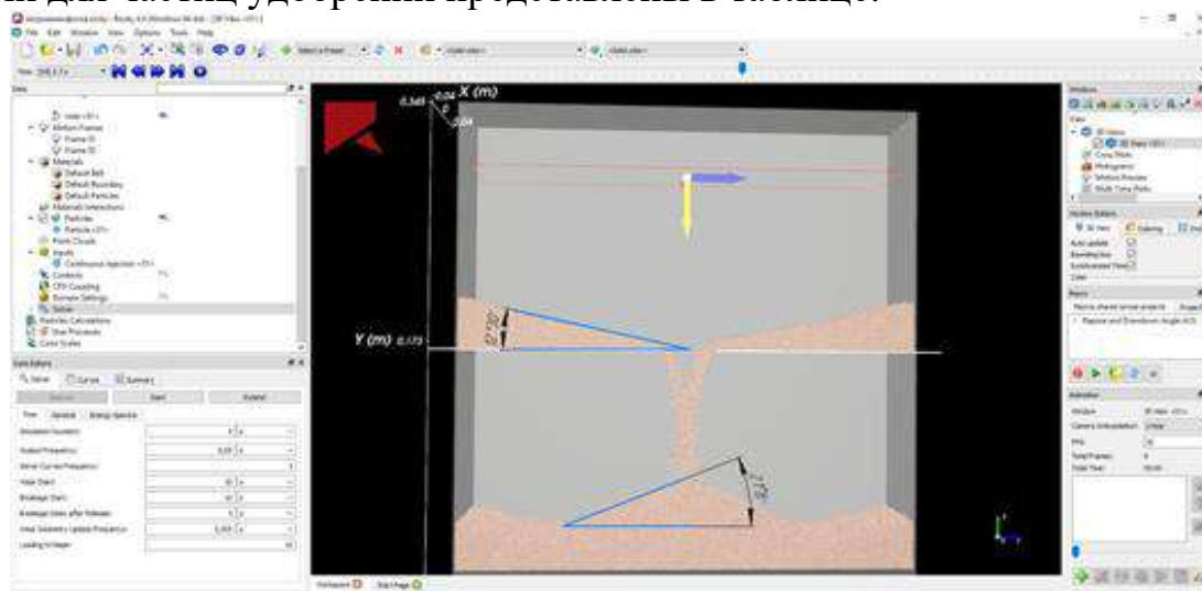
Рис. 1 Цифровой двойник измерения угла обрушения в программе ROCKY DEM
