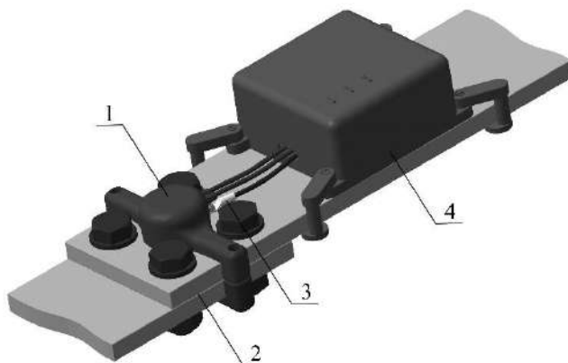
Рис. 2 Размещение автономного устройства акустической эмиссии плоскостного контакта шин
